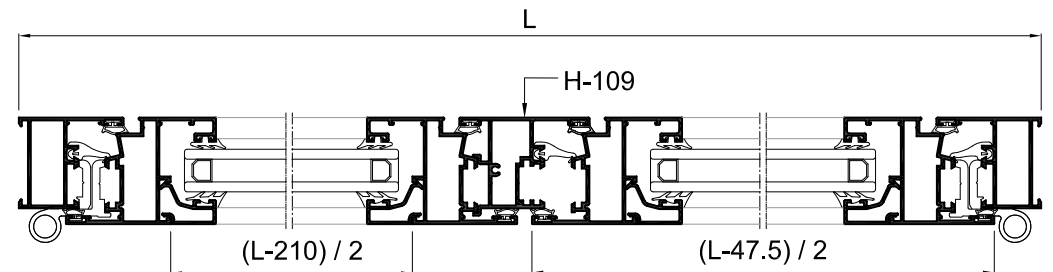
Sección A-A'
